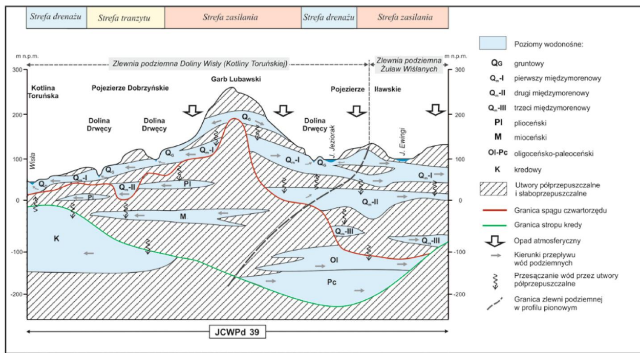
Rysunek 14. Schemat przepływu wód podziemnych w JCWPd nr 39
