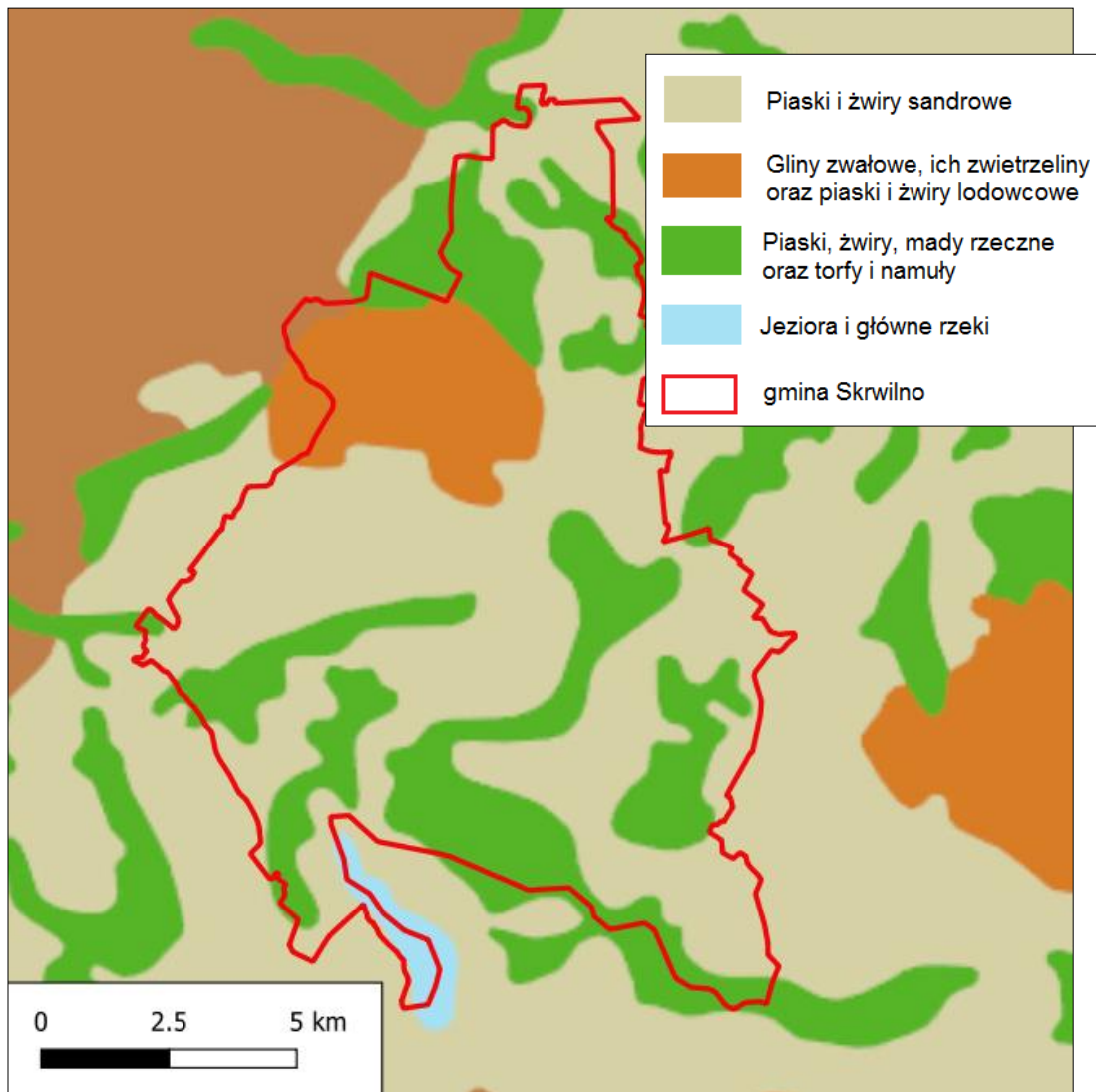
Rysunek 8. Powierzchniowe utwory geologiczne na obszarze opracowania
